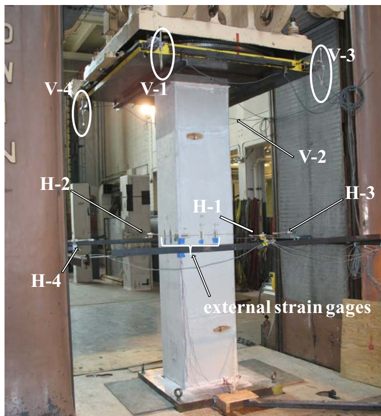
Fig. 2: Test setup
